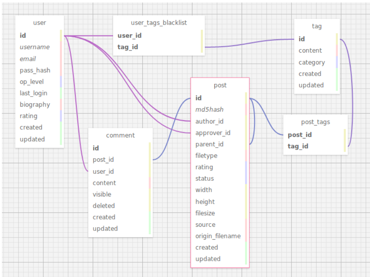
Obrázek 2: ER diagram
